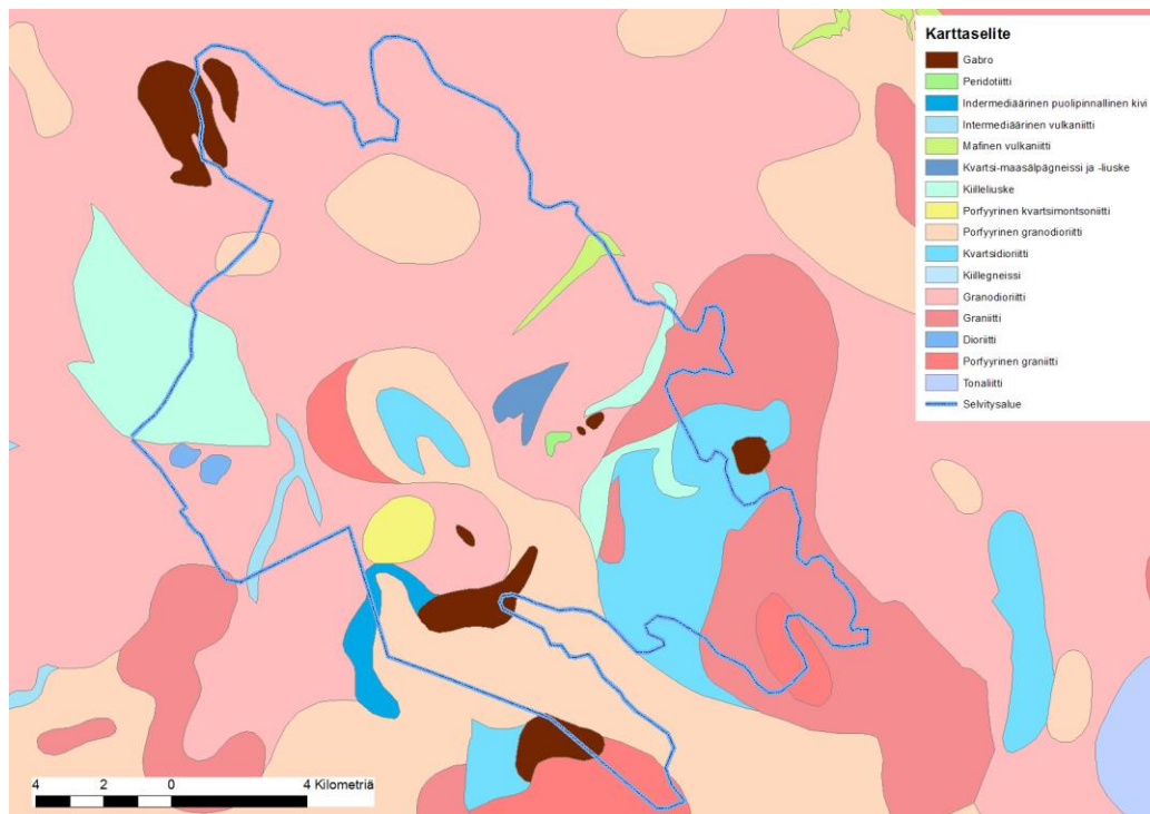
Kuva 3. Kallioperä (© GTK 2015).
