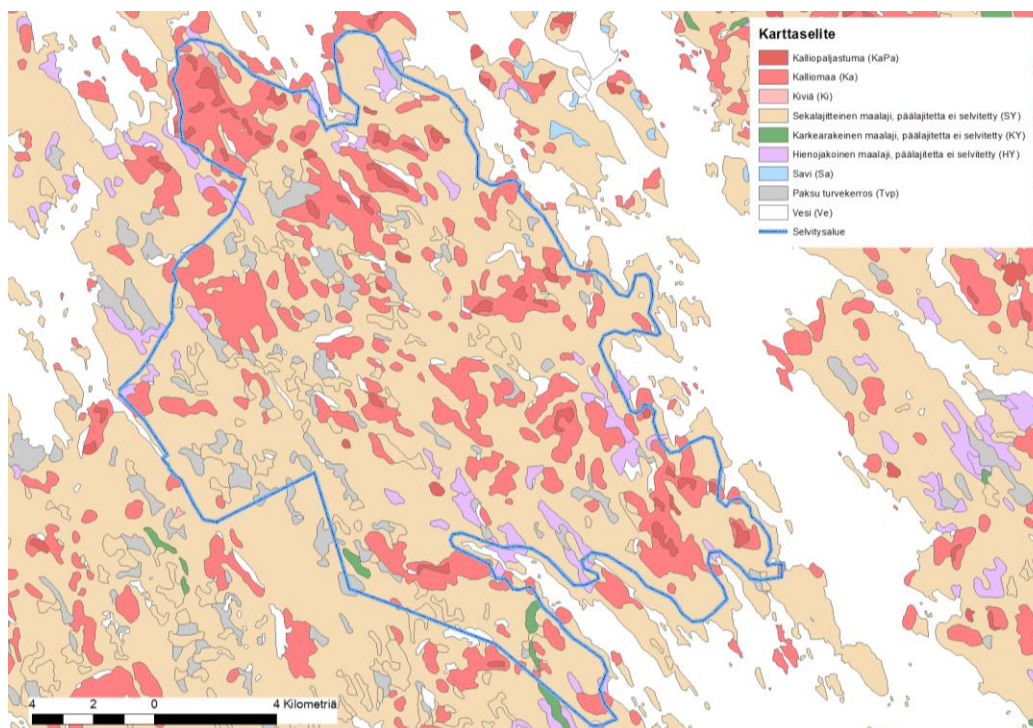
Kuva 4. Maaperä (© GTK 2015).
