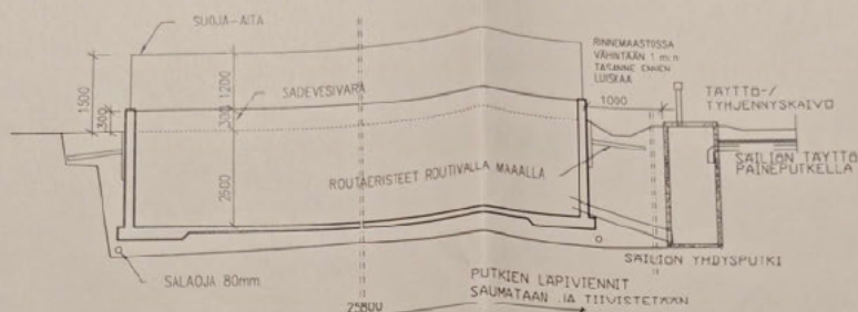
LEIKKAUS 1:100
