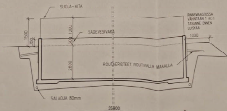
LEIKKAUS 1:100
